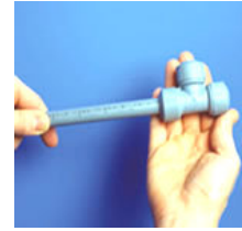
Insertar el tubo en la pieza. Girar un poco y presionar hasta el fondo. Para finalizar, pegar un fuerte tirón del tubo.
