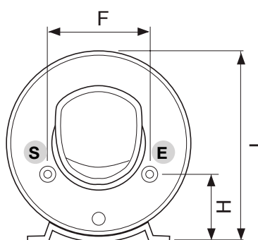
Vista V sólo para dimensiones
